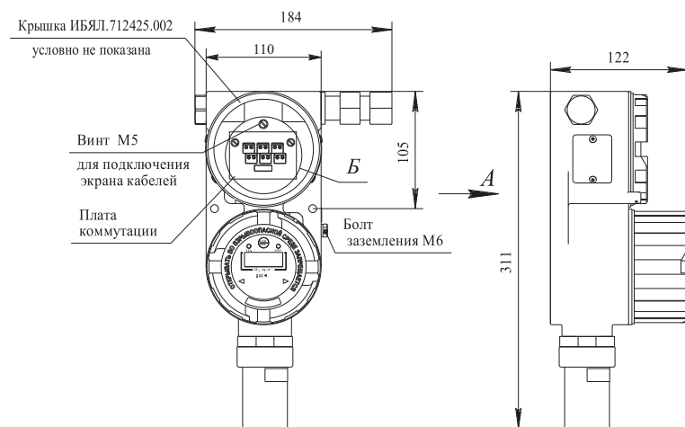
в) газоанализаторы ДАХ-М-05/-05Х/-05ХН/-06/-06ТР/-06ТРХ/-06ТРХН
