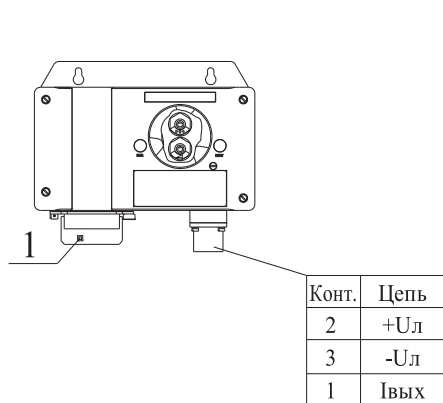
б) газоанализаторы ДАХ-М-03/-04
