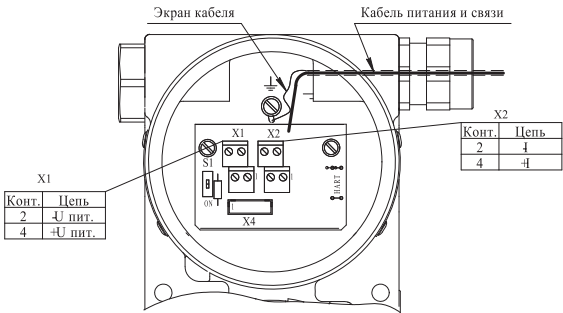
Рисунок И.2 - Монтажный чертеж газоанализаторов ДАХ-М-05Х/-06ТРХ/-08Х/-08ТРХ
