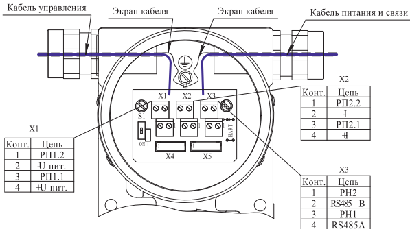
Рисунок И.2 - Монтажный чертеж газоанализаторов ДАХ-М-05Х/-06ТРХ/-08Х/-08ТРХ
