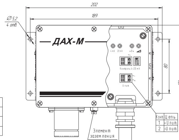
г) газоанализатор ДАХ-М-07/-07Н
