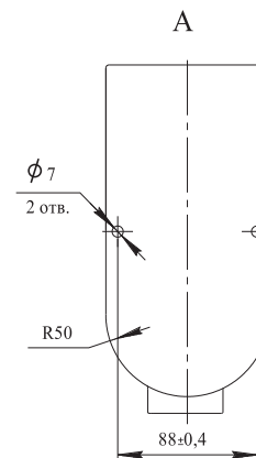
в) газоанализаторы ДАХ-М-05/-05Х/-05ХН/-06/-06ТР/-06ТРХ/-06ТРХН
