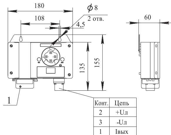
а) газоанализаторы ДАХ-М-01
